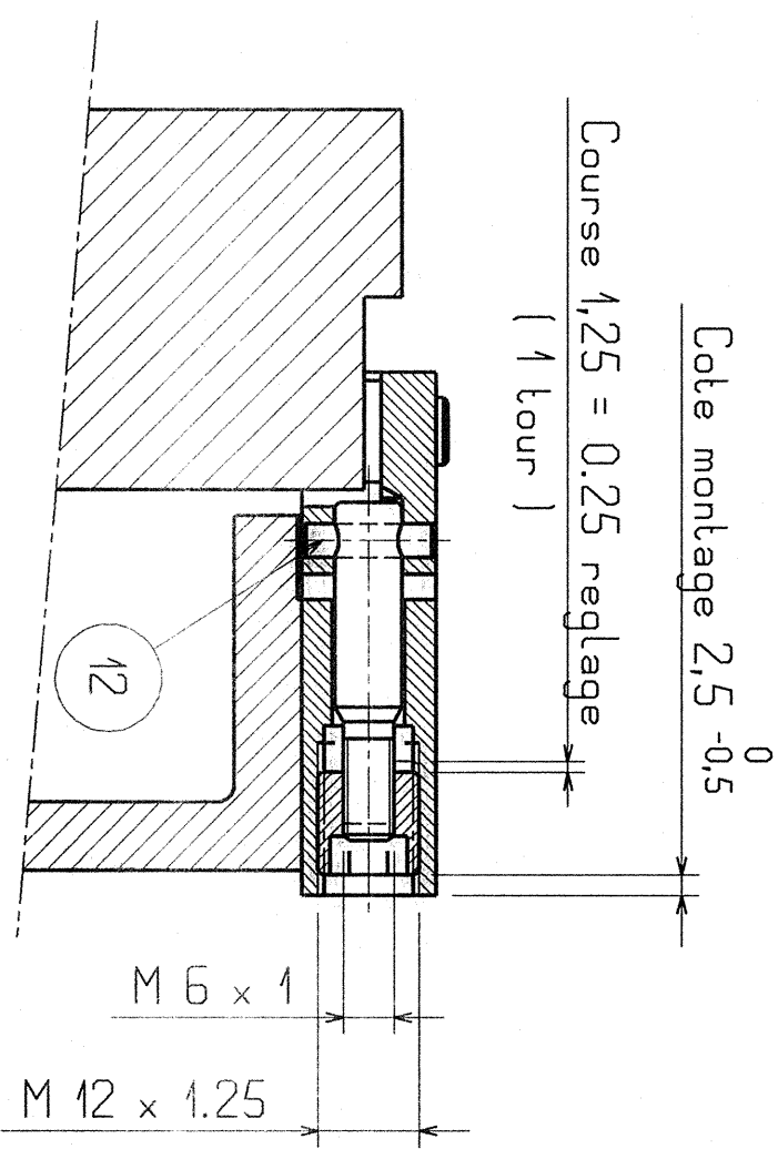
Coupe BB
