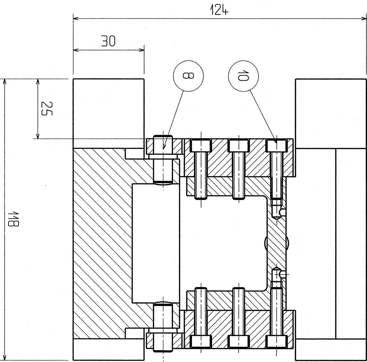
Coupe AA
